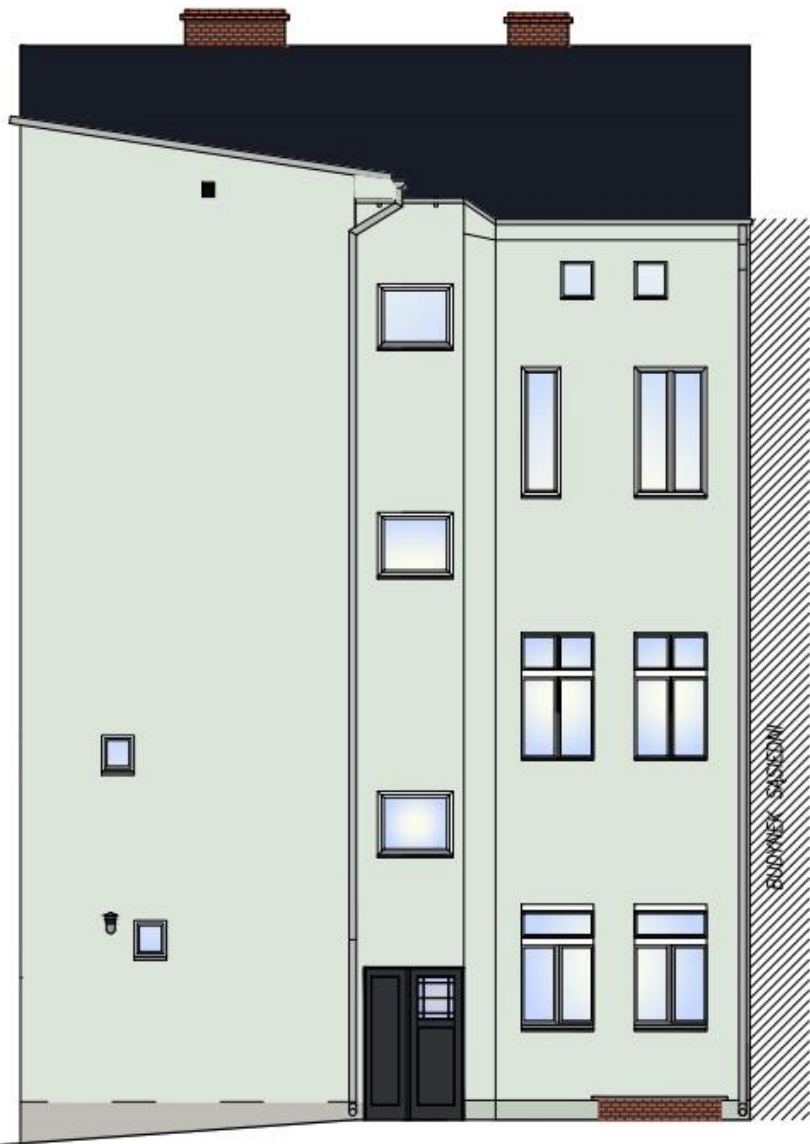
ELEWACJA PÓŁNOCNO-WSCHODNIA
